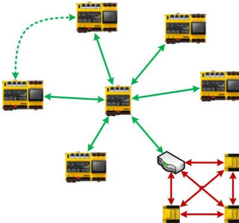
Abbildung 4 Hub-und-Spoke-Topologie von BACnet/SC. Während die BACnet/SC-Kommunikation im Hub zentralisiert wird, erfolgt die BACnet/IP-Kommunikation zwischen den einzelnen Stationen («Station to Station») oder mittels Broadcasting.
