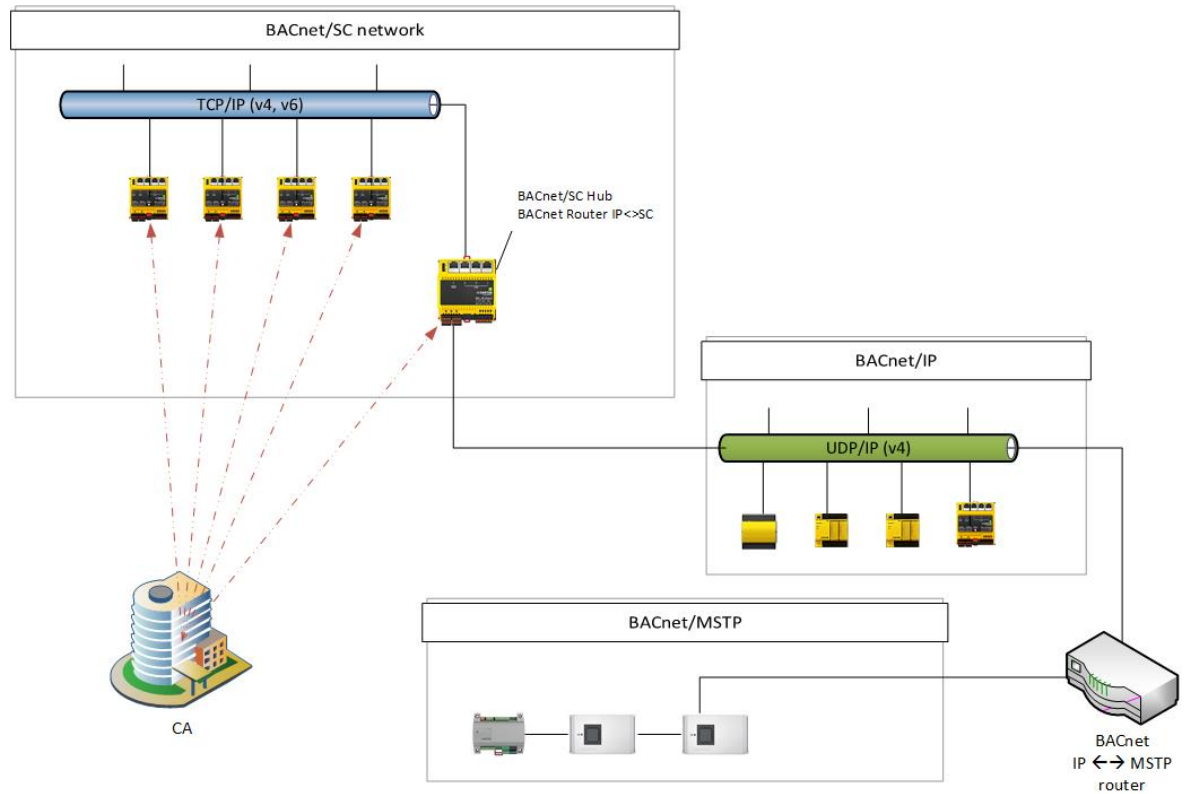
Abbildung 3 Verschiedene BACnet-Netzwerke und -Geräte
