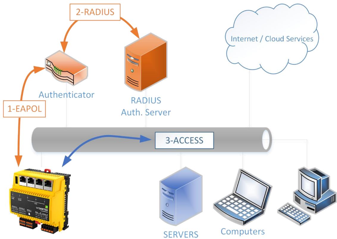
Figure 7 802.1X Topologie und Protokolle 1. Zugang verlangen 2. Identitätsprüfung 3. Zugang an weitere Ressourcen zugelassen
