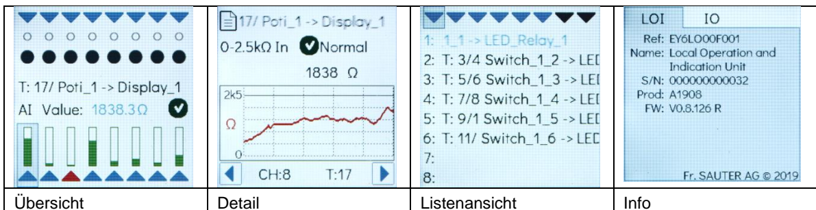
Abbildung 2 Grafische Benutzeroberfläche
