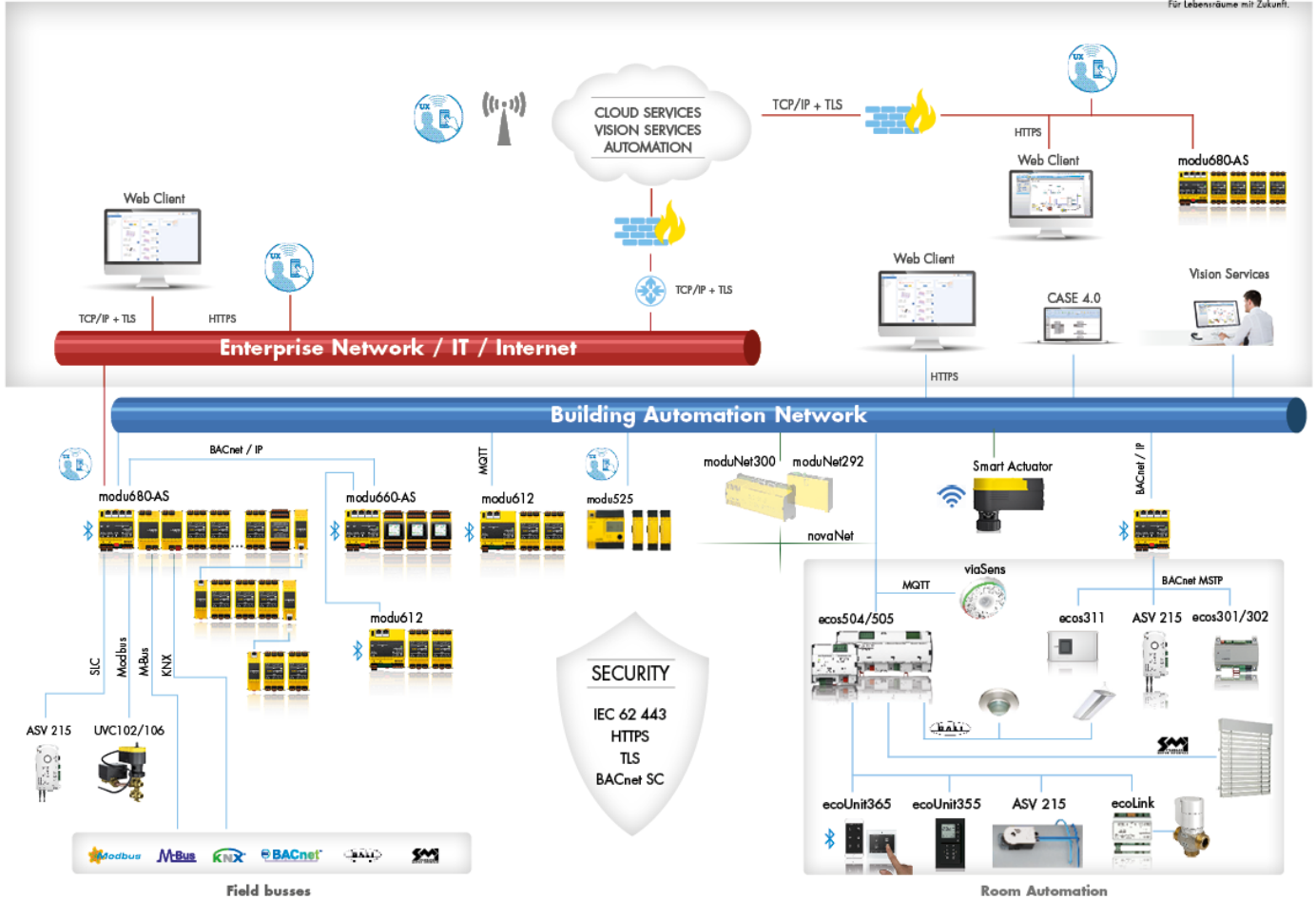
SAUTER modulo 6 Topology
